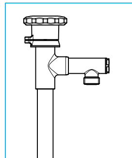
Typ P1000-RGL (abschließbar)
